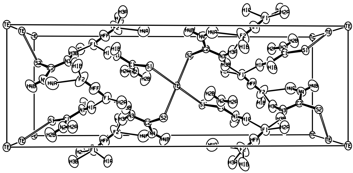
TETRATHIOUREA-TELLURIUM (II) DI (HYDROGENFLUORIDE)
